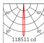
XP-E2 7° 2700K
